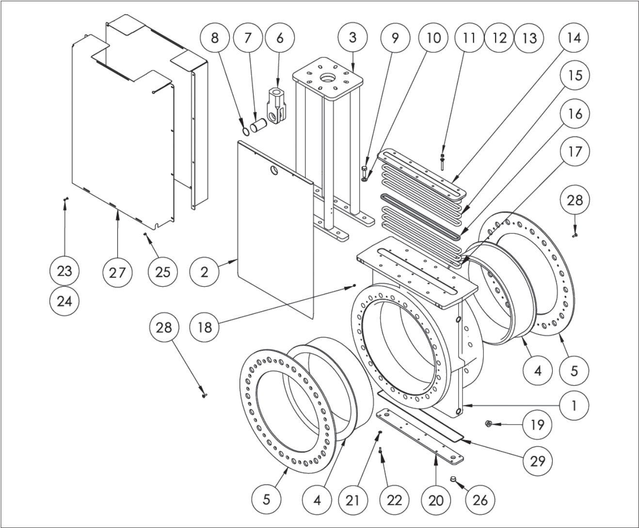
SKH 分解图
