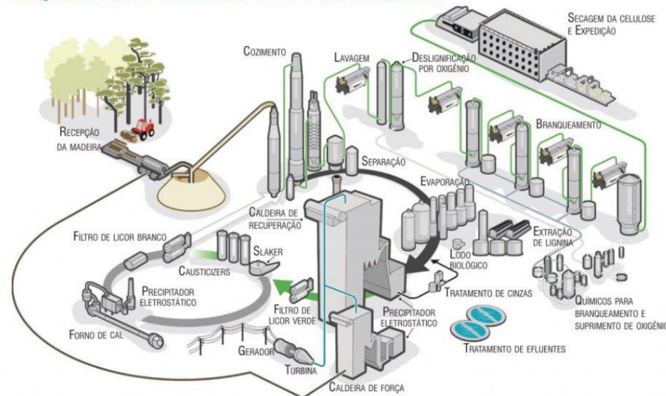
ESQUEMA DO PROCESSO KRAFT DE CELULOSE
